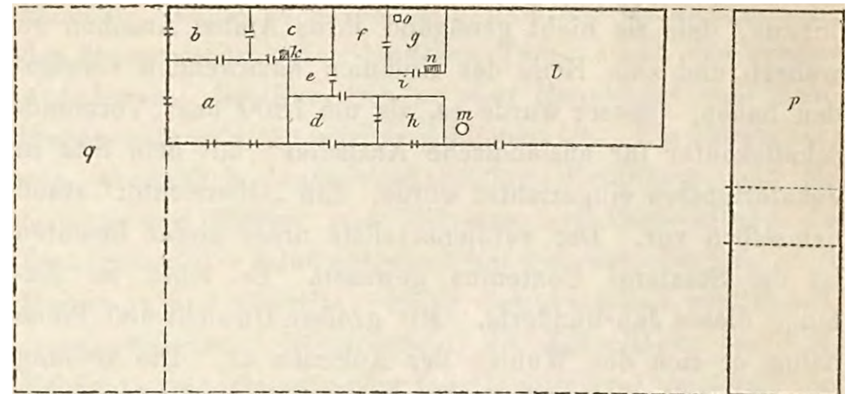
a Grosse Stube e Küche i Gang zum Stall n Bodentreppe b Eckstube f Hinterflur k Grosser Ofen o Kellerthür c Kleine Stube g Speisekammer l Stall p Scheune d Vorflur h Sommerstube m Brunnen q Vorgarten
